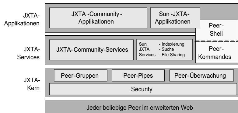
Abb. 3: Die JXTA-Architektur
