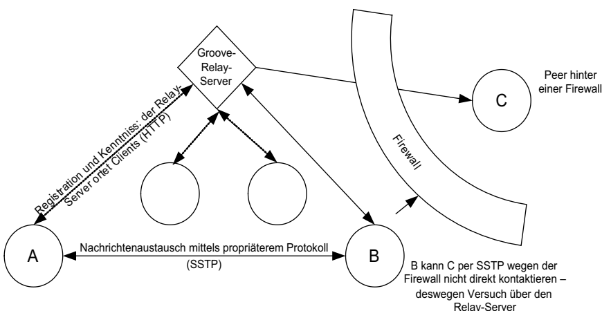
Abb. 4: Groove-Anwendungsszenario
